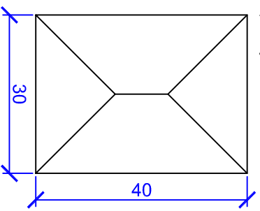
půdorys
