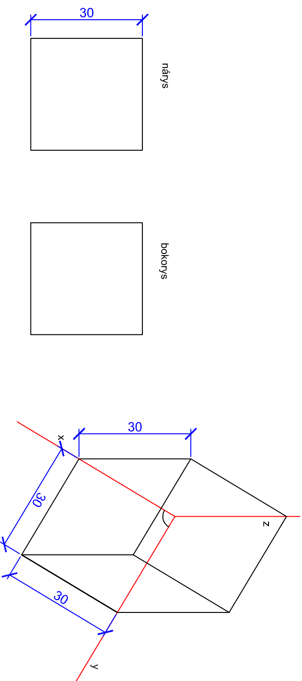
KP - tzv. vojenská perspektiva
