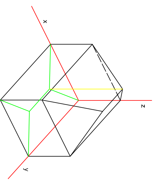
Pravouhlá axonometrie - trimetrie
